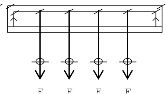
1x4 4 st punktlaster
